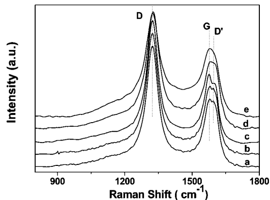
Figure 4. Raman spectra of (a) p-MWNTs, (b) MWNT-OH, (c) MWNT-NH 2 , (d) MWNT-COOH, and (e) MWNT-Br.
